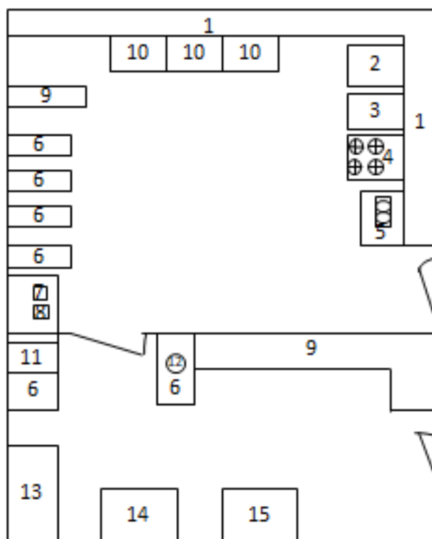
Рис. 2.5 – План кондитерского цеха
